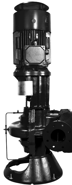
Grundfos LSV pump
